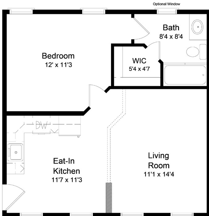
In-Law Suite #3- 576 Sq Ft
